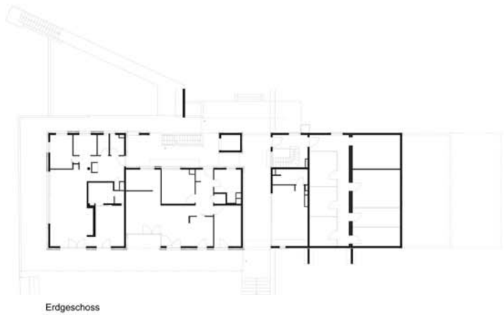
Erdgeschoss
